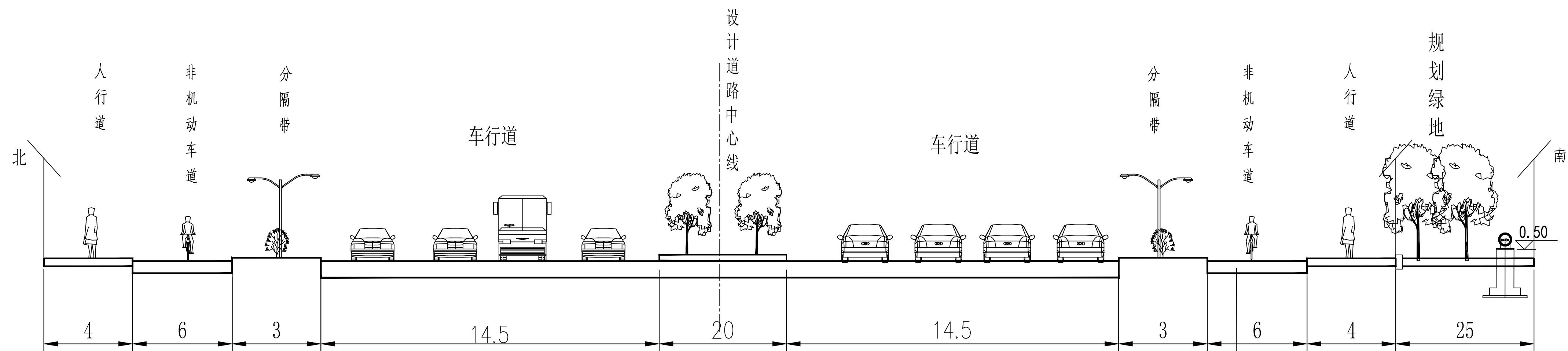
槐安东路横断面图 (燕山大街—泰山街)
