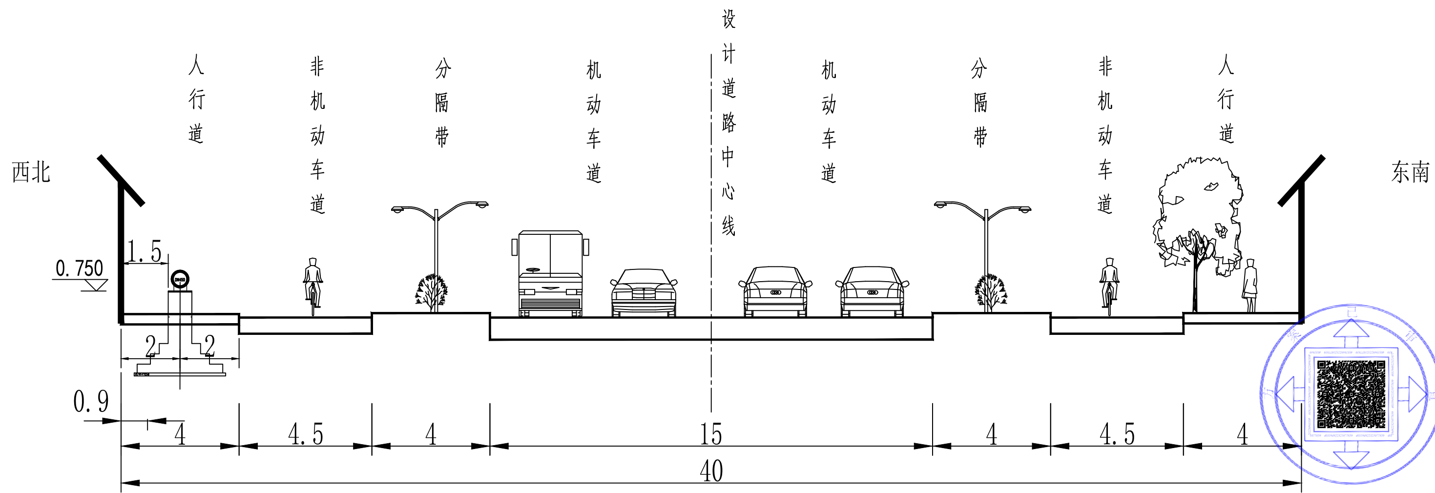
郅马路横断面图 (太行西街-秦岭大街)
