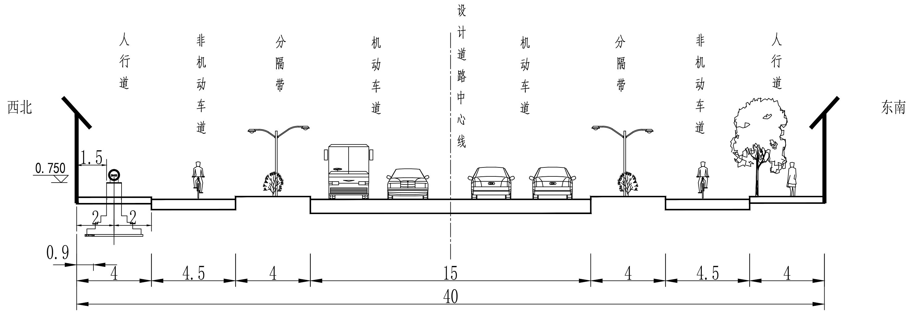
郅马路横断面图 (太行南大街-太行西街)
