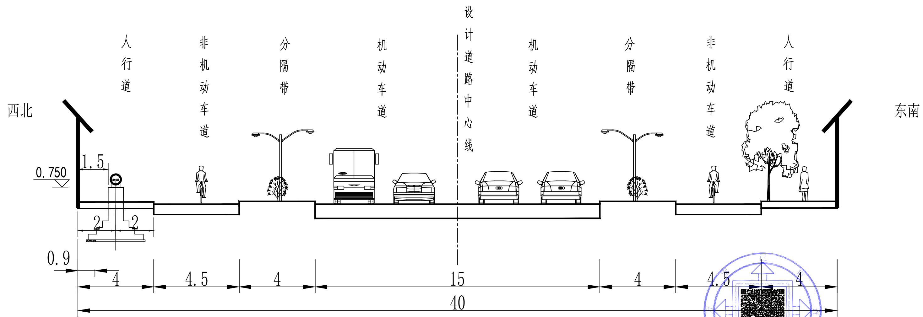
邻马路横断面图 (苍岩街-昆仑大街)
