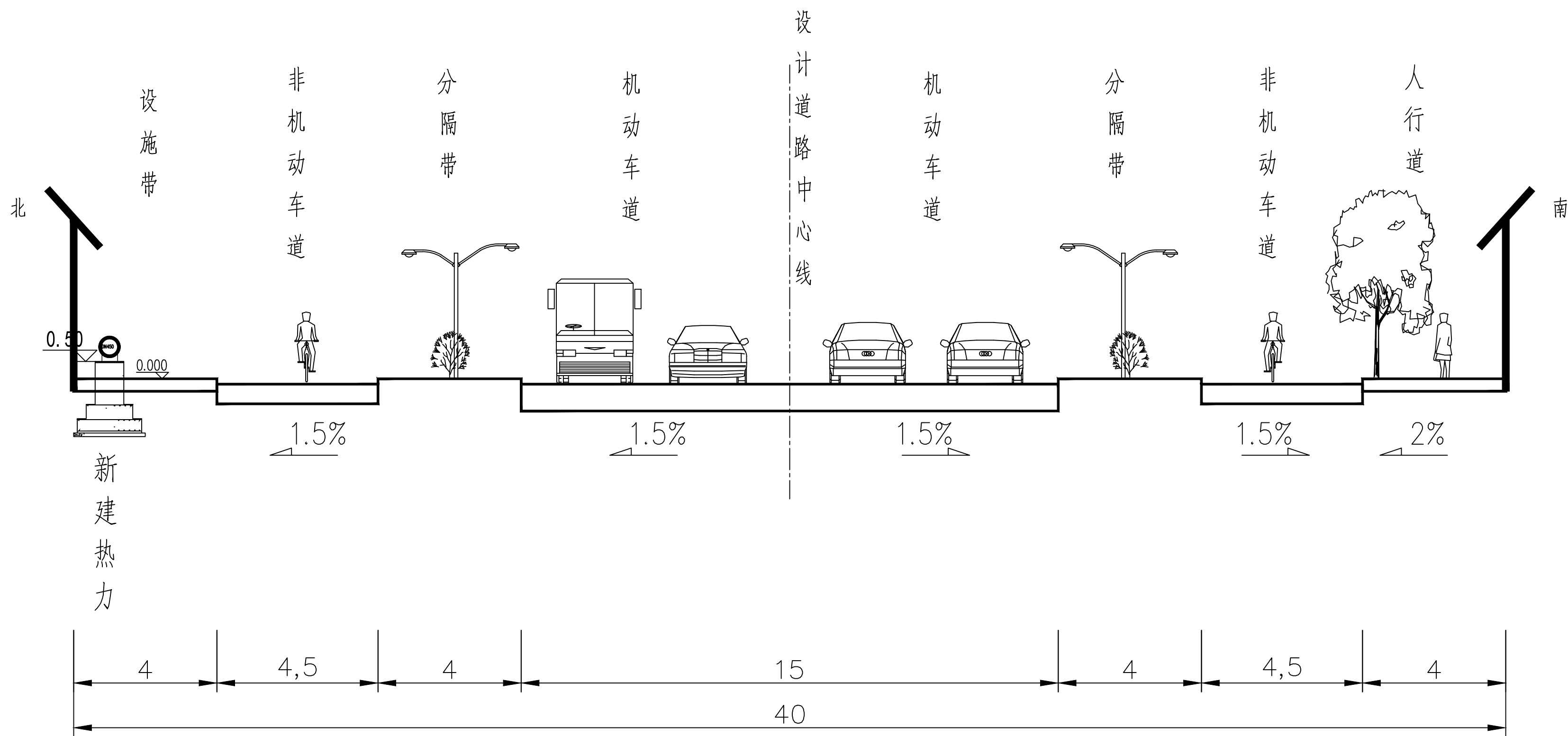
郅马路横断面图 (段干路—燕山大街)
