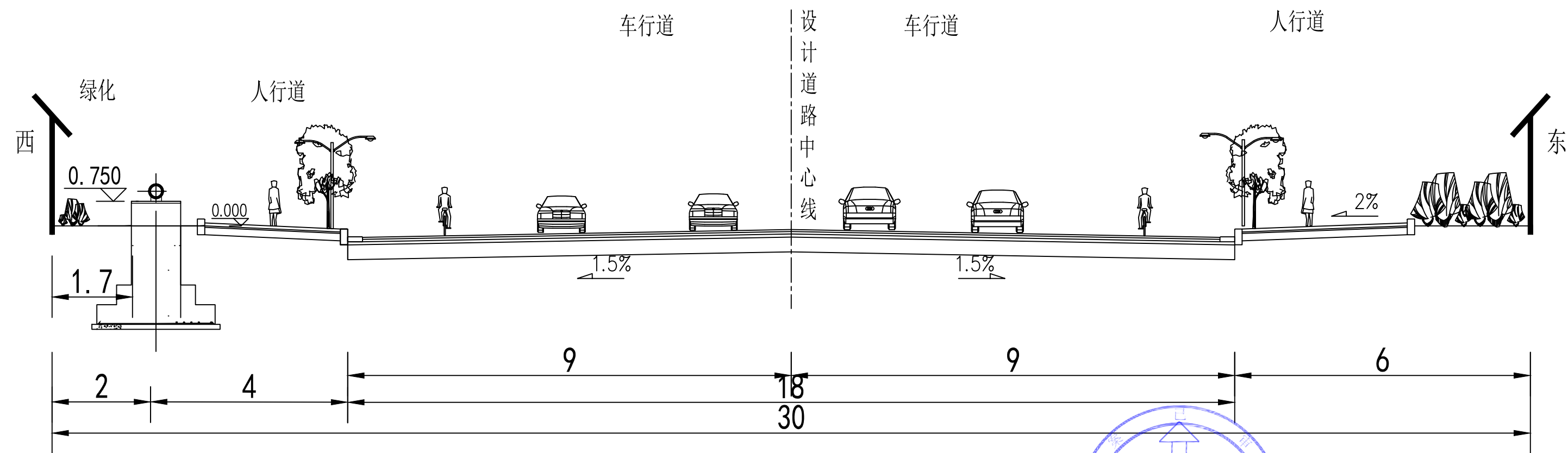
苍岩街(鄗马路南)横断面
