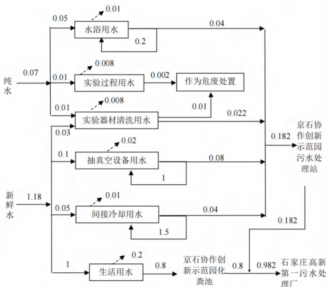
图 2-1 本项目给排水平衡图 单位: m³/d
