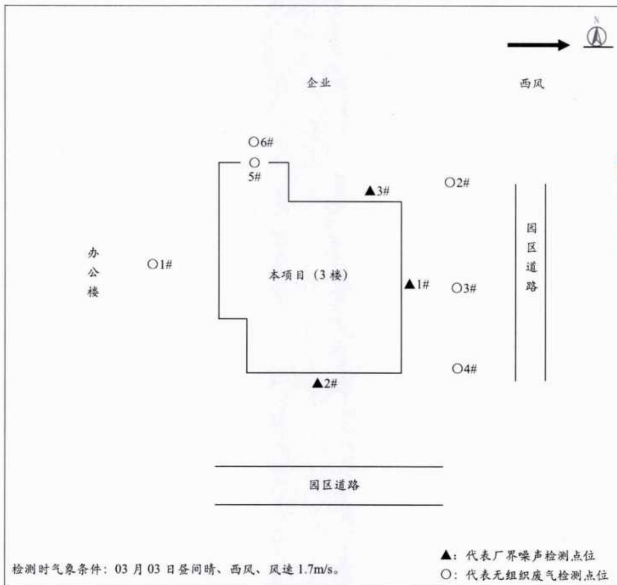
附图：厂界噪声及无组织废气检测点位示意图（续）
